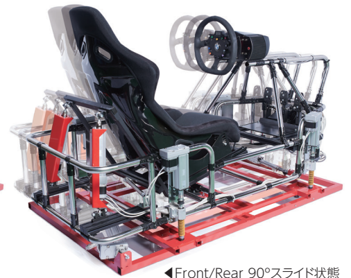
◀Front/Rear 90°スライド状態
