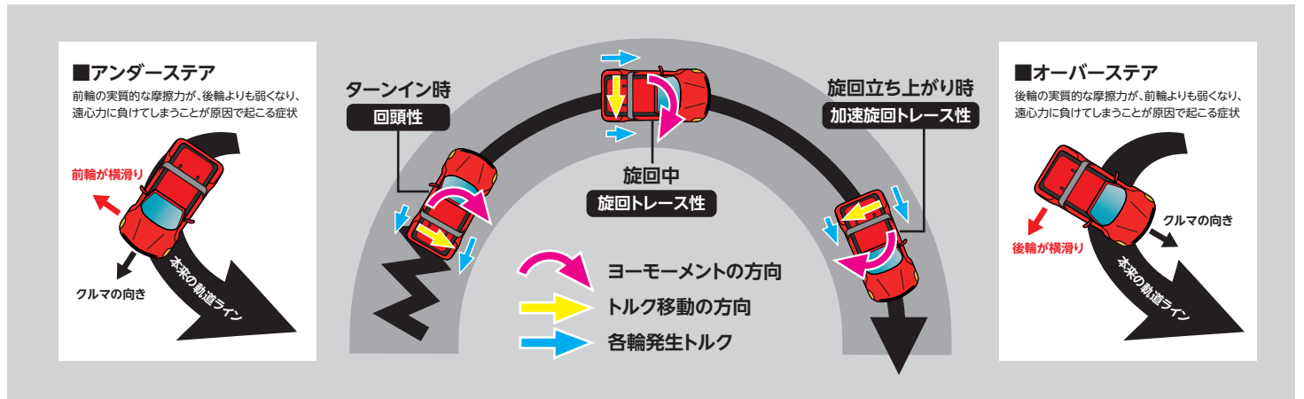
◀Frontスライド状態
